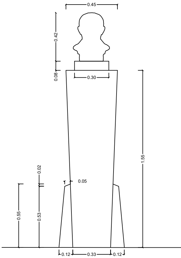
ALZADO
