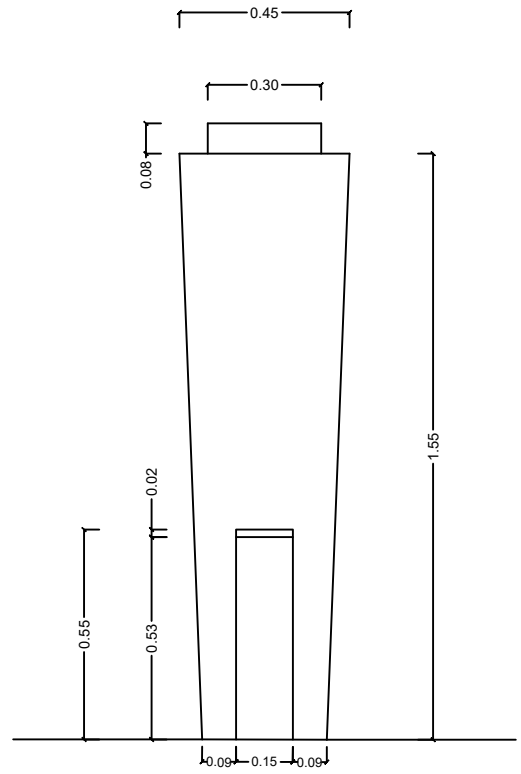
ALZADO LATERAL
